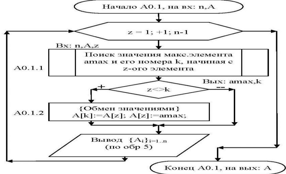
Рис. Блок-схемы алгоритма для задачи Extremum
